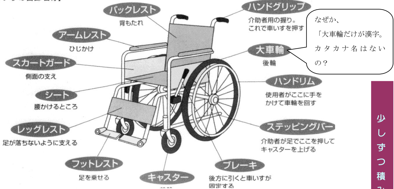
【車いすの各部名称】
